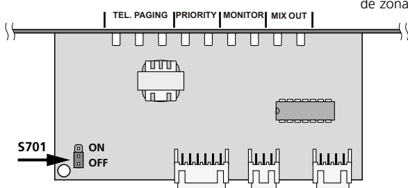
Jumper S701 Prioridad para las entradas CH 1 y TEL PAGING
